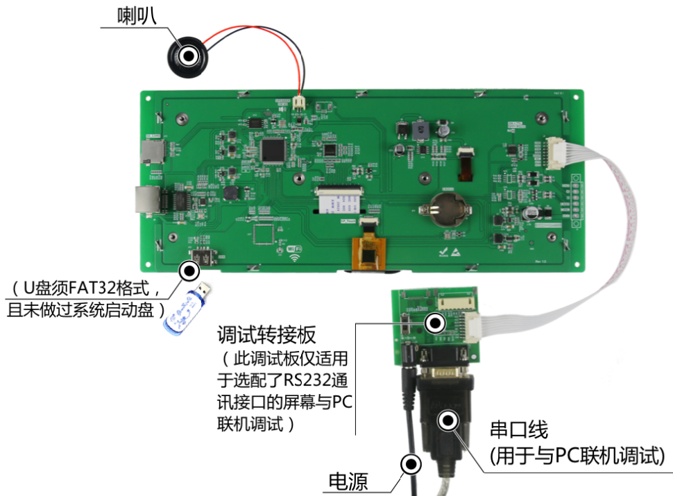
图 1-4 调试工具
