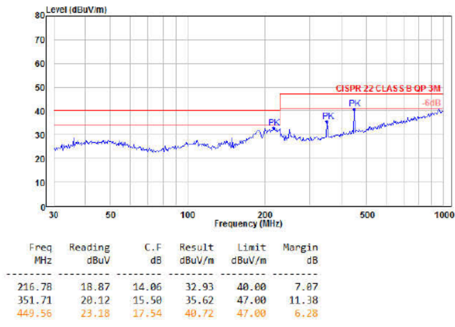
图 3-6 辐射测试水平方向
