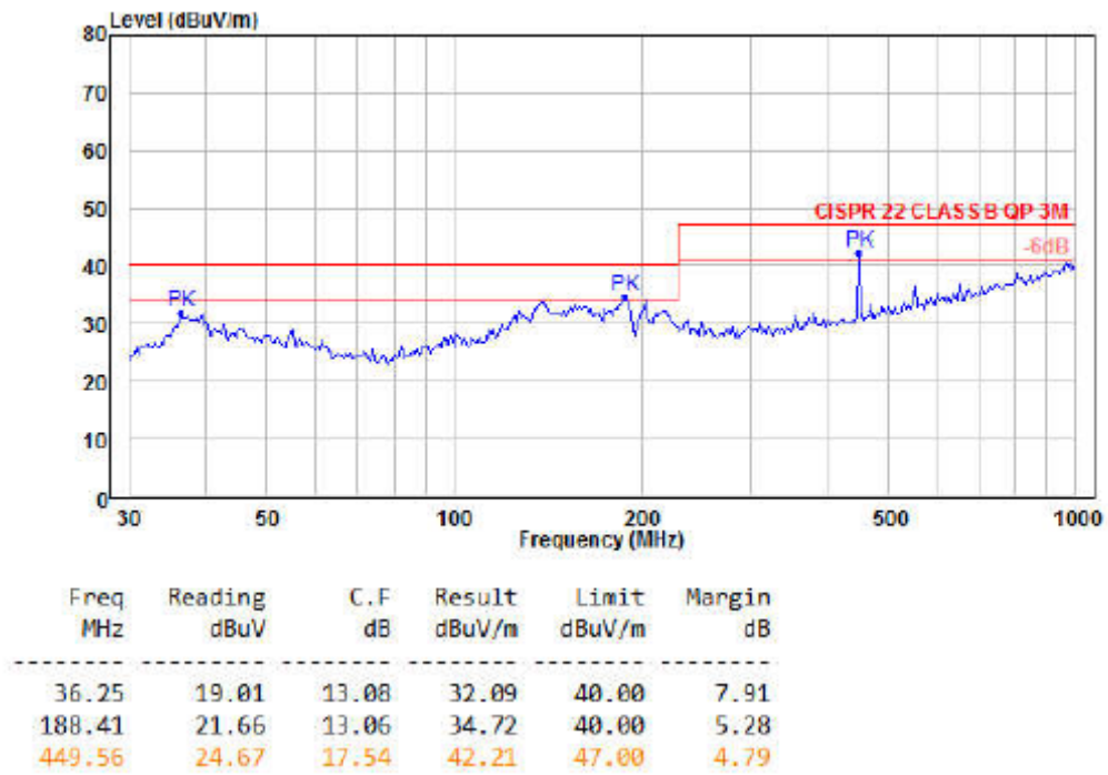
图 3-7 辐射测试垂直方向
