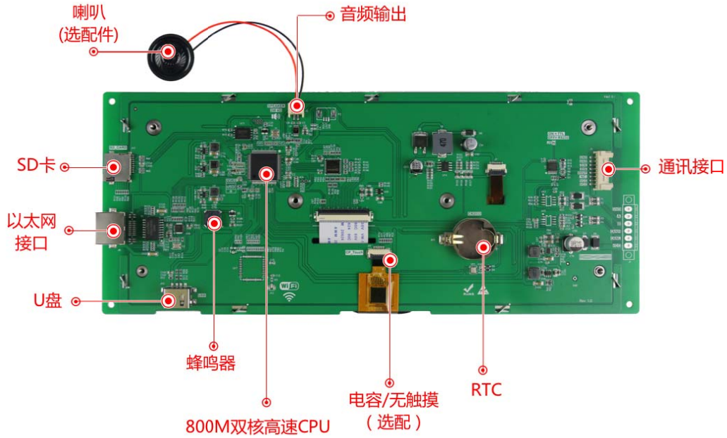
图 1-3 硬件配置图
